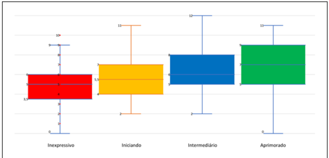
Figura 27 - Distribuição dos valores de iBackup em cada estágio de capacidade em gestão de SegInfo.
